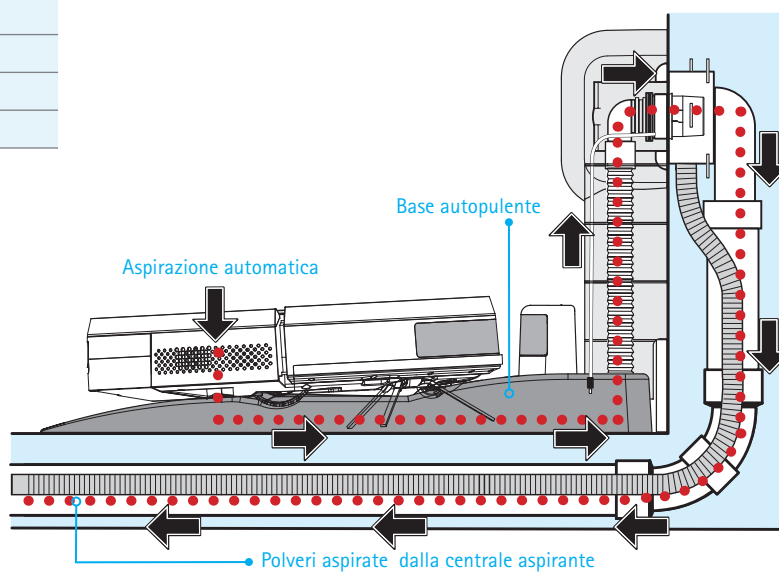
Schema del flusso polveri da ROBÒ alla base autopulente
